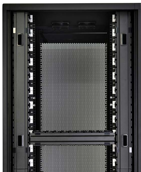
19" 加寬型機櫃(加裝手指線槽示意圖)
