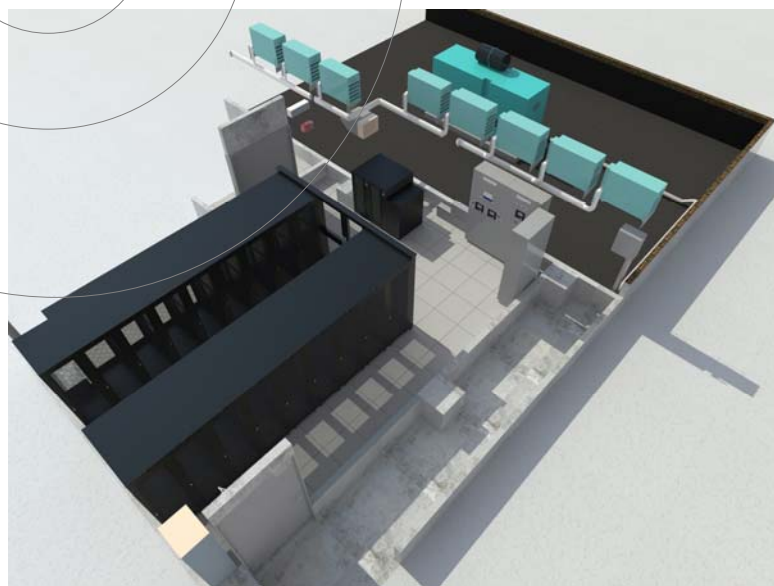
節能冷熱走道封閉規劃設計
